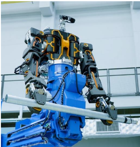
零式人機 ver. 2.0（実機）
