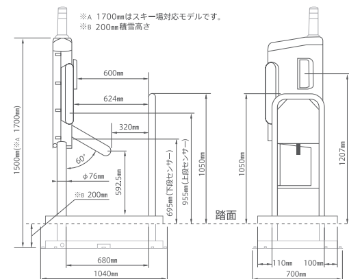
正面図
