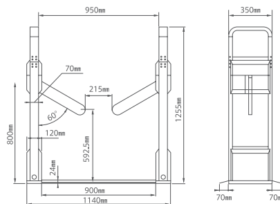
正面図
